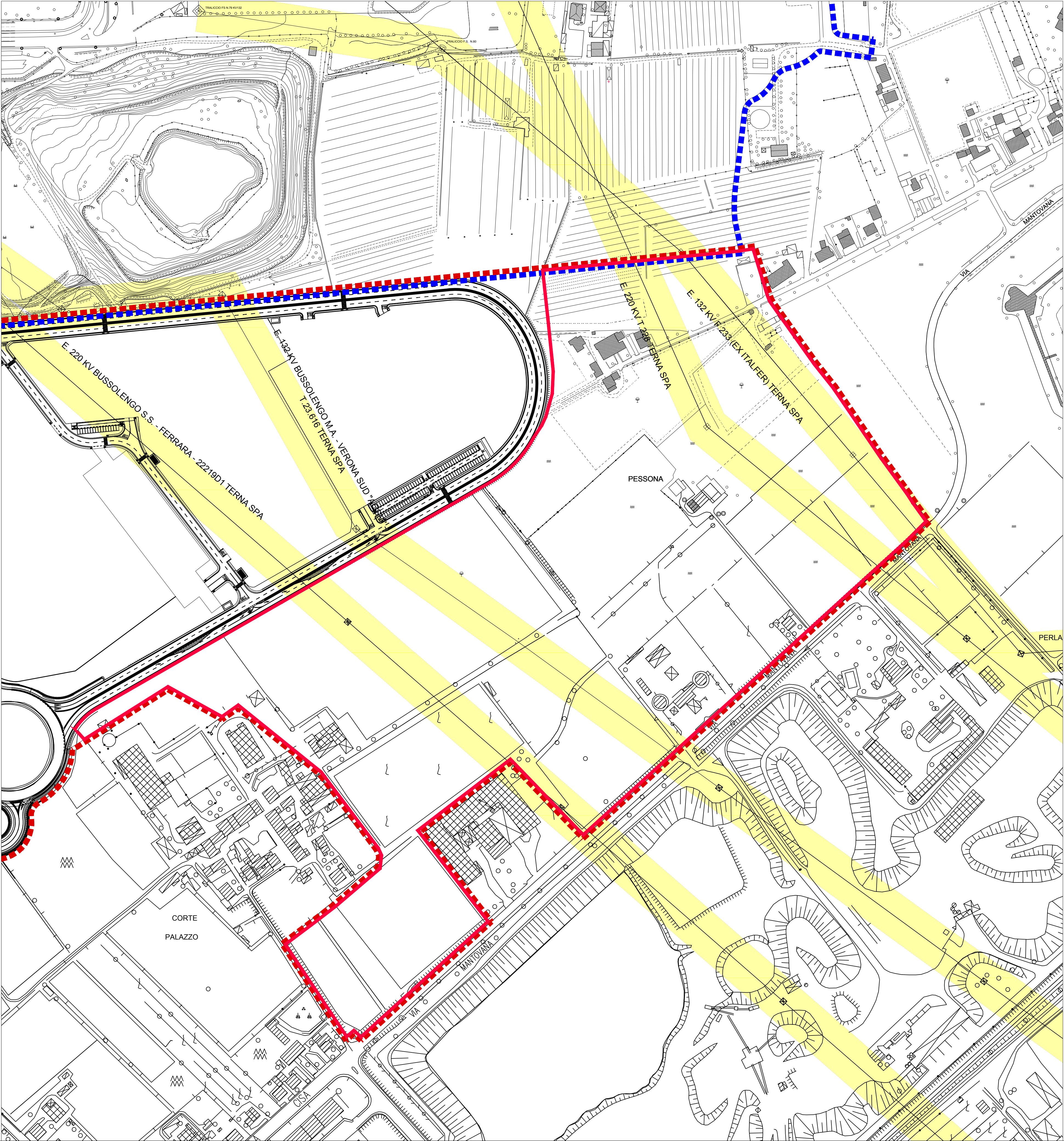
Tav. 3 Ricognizione dei vincoli gravanti sull'area
